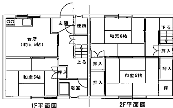
1F平面図
