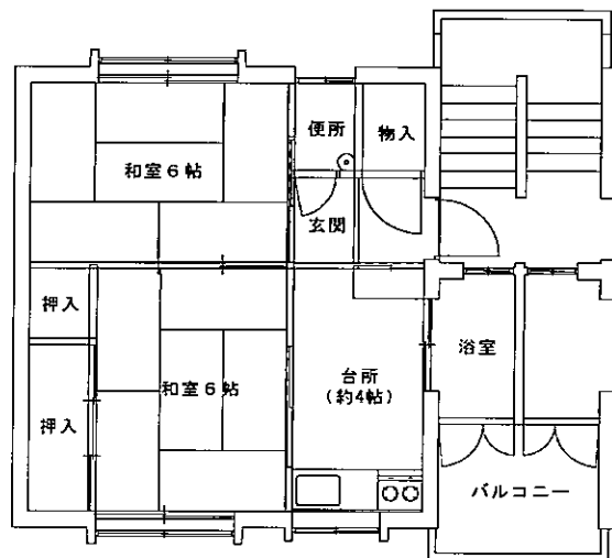
当新田市営住宅（2DK中耐タイプ）
