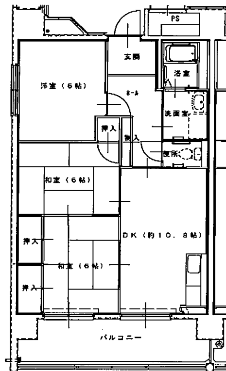
芳田市営住宅（3DKタイプ）
