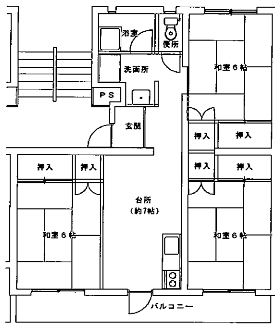
山田西・山田B市営住宅（3DKタイプ） 久保A・久保C・宿毛東・宿毛南市営住宅
