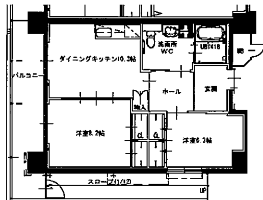
さくら住座（下肢住宅2DK）
