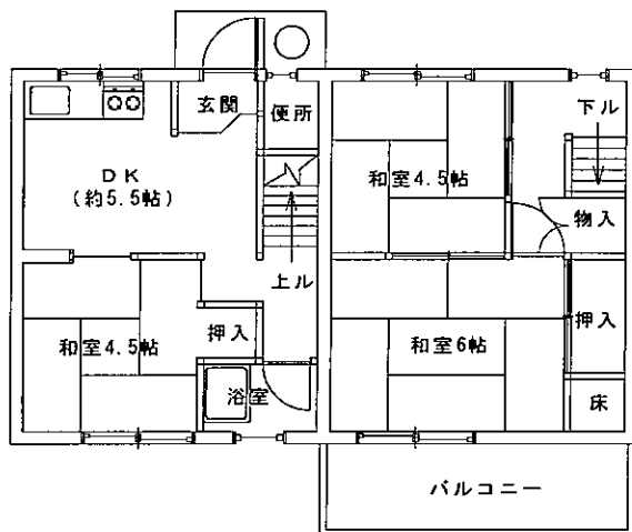
1F平面図
