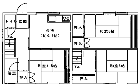
1F平面図
